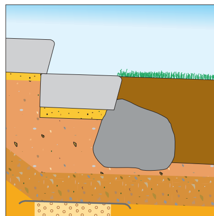
Eksempel på kantsikring af nederste trin.
