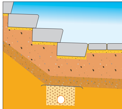
Elementtrappe med effektivt dræn under nederste trin.
